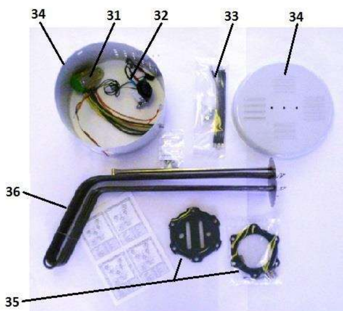
KIT 15/30 kW pour bride Ø 110mm AJ165/166
